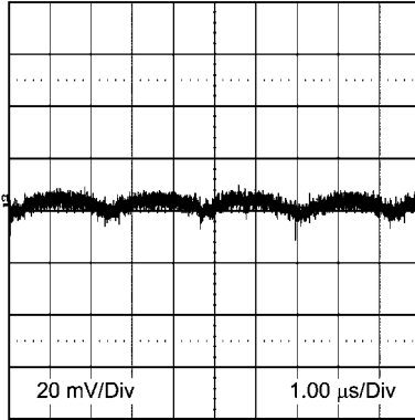
Output Ripple 24V_{IN} 3.3V_O 2A , BW = 200\text{ MHz}
